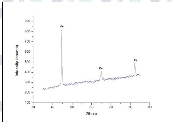
Gambar 4. Grafik Hasil XRD Coperrized-AISI 1006
