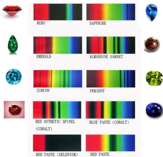
Gambar 2. 5 Contoh spektrum warna dari setiap batu mulia yang berbeda [17]
