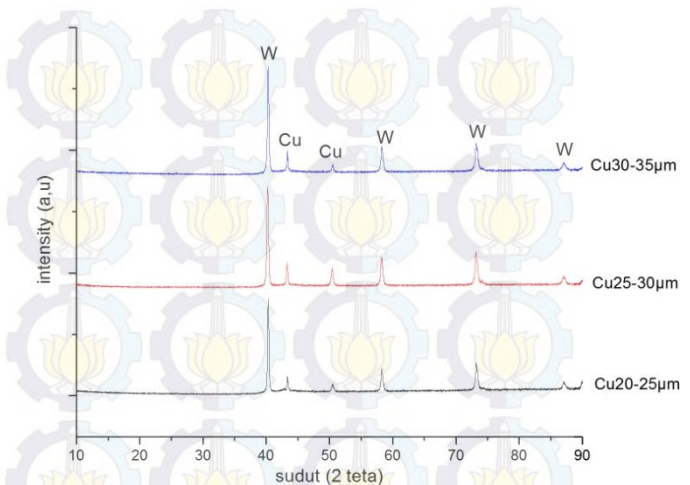
Gambar 4.6 Grafik XRD pada temperatur 1100 0 C
