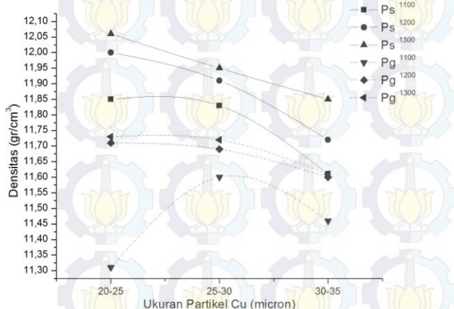
Gambar 2. Pengaruh ukuran partikel Cu terhadap green dan sinter density
