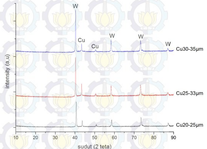
Gambar 4.7 Grafik XRD pada temperatur 1200 0 C
