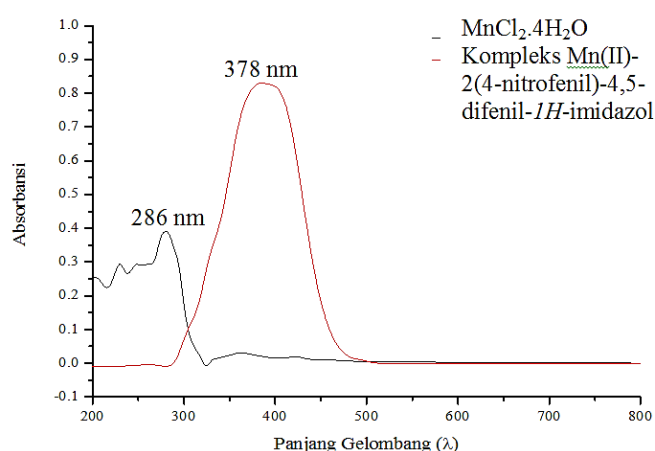
Gambar 2. Hasil Pengukuran Panjang Gelombang Maksimal \text{MnCl}_2 \cdot 4\text{H}_2\text{O} dan Kompleks Mn(II)-2(4-nitrofenil)-4,5-difenil-1 H -imidazol
