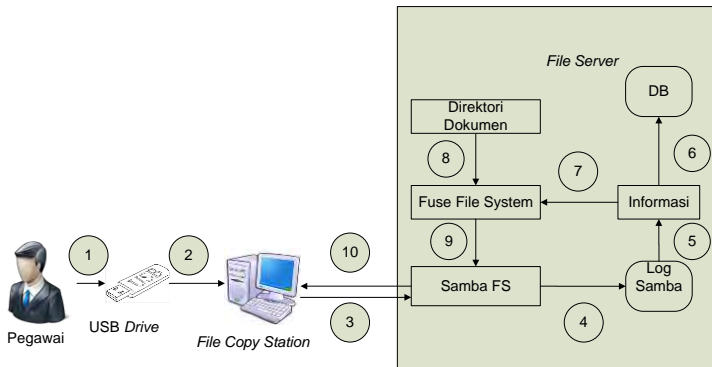
Gambar 3.1 Arsitektur umum sistem
