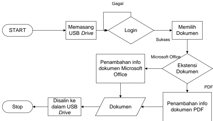
Gambar 3.4 Diagram alir penyalinan dokumen
