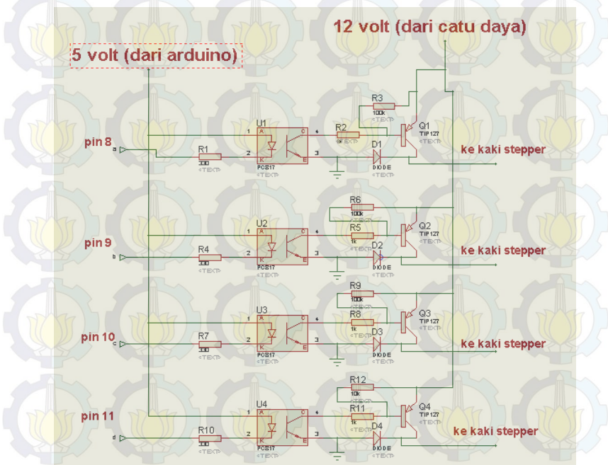
Gambar 3.5 Driver untuk Stepper
