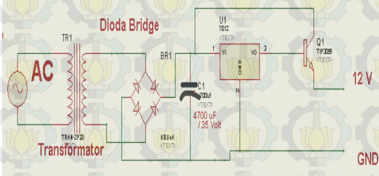
Gambar 3.3 Rangkaian Catu daya
