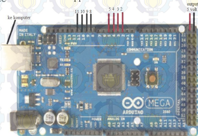
Gambar 3.4 letak pin Arduino yang digunakan
