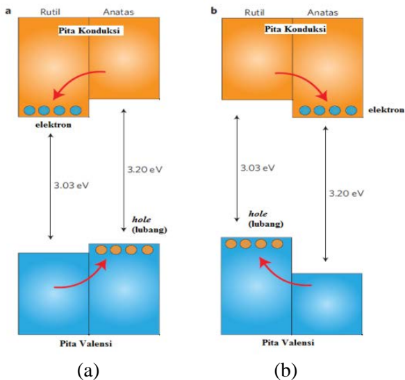
Gambar 2.8 Gambar celah energi yang dimiliki oleh anatase (a) dan rutile (b)
