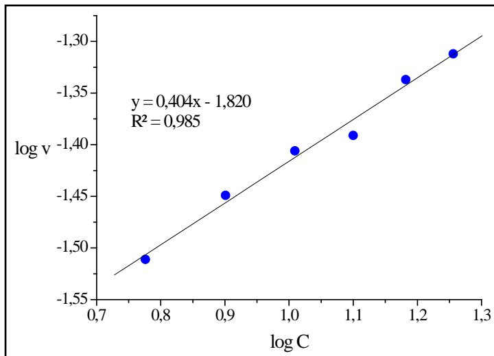
Gambar 4.8 Grafik plot antara log \nu dan log C, pada konsentrasi awal 20 ppm dan pH 7
