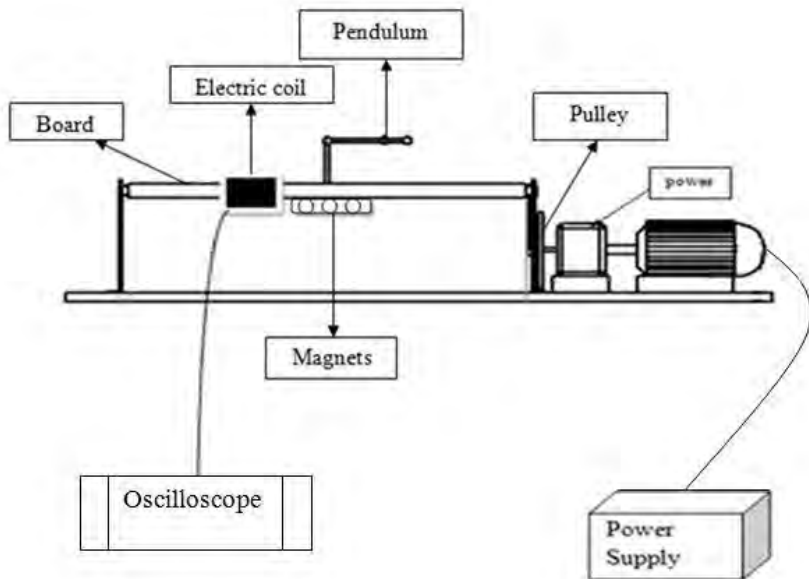
Gambar 3.16 Skema Percobaan
