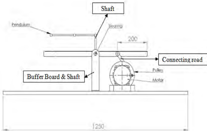
Gambar 3.3. Pemodelan 2D Mekanisme (Tampak Samping)
