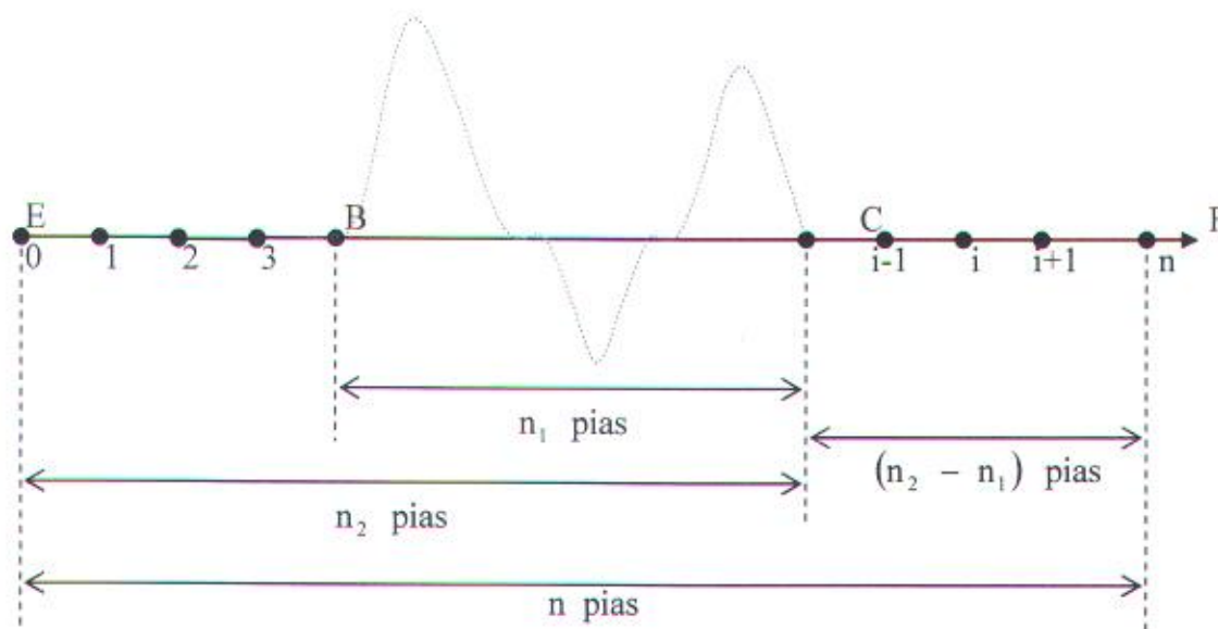
Gambar 3.4. Diagram titik-titik pias pada dasar saluran
