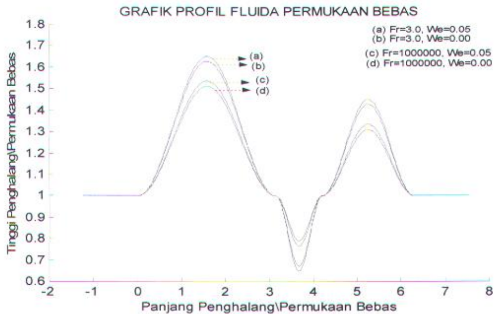
Gambar 4.5. Profil permukaan bebas dengan variasi bilangan Fr=3.0 dan Fr=10^6 , dengan bilangan We=0.00 dan We=0.05
