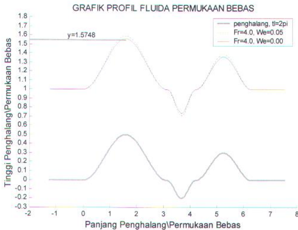
Gambar 4.2. Profil permukaan bebas dengan bilangan Fr=4.0 , dengan variasi bilangan We=0.05 , We=0.00 .
