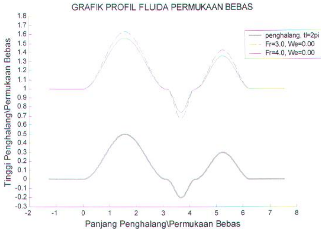
Gambar 4.4. Profil permukaan bebas dengan variasi bilangan Fr=3.0 dan Fr = 4.0 , dengan bilangan We=0.00 .
