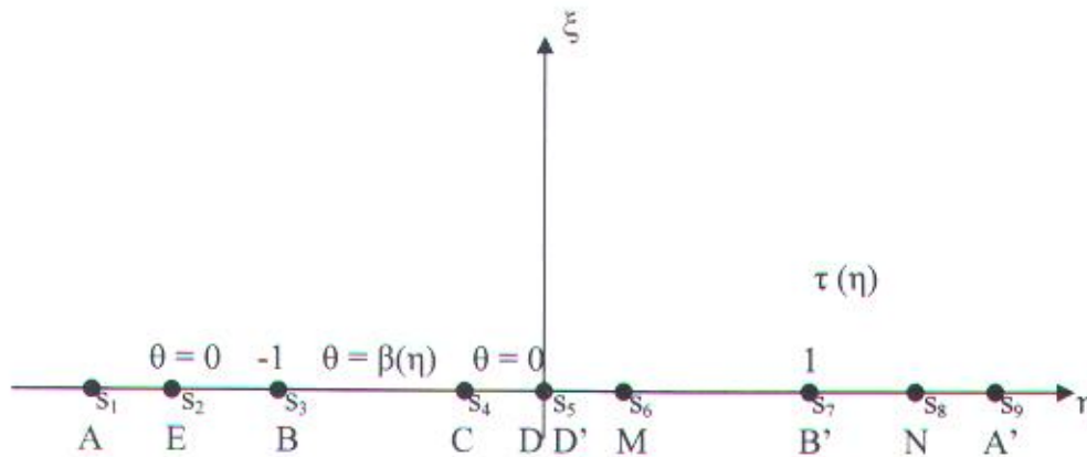
Gambar 3.3. Pemetaan bidang- \omega ke bidang paruh- t .
