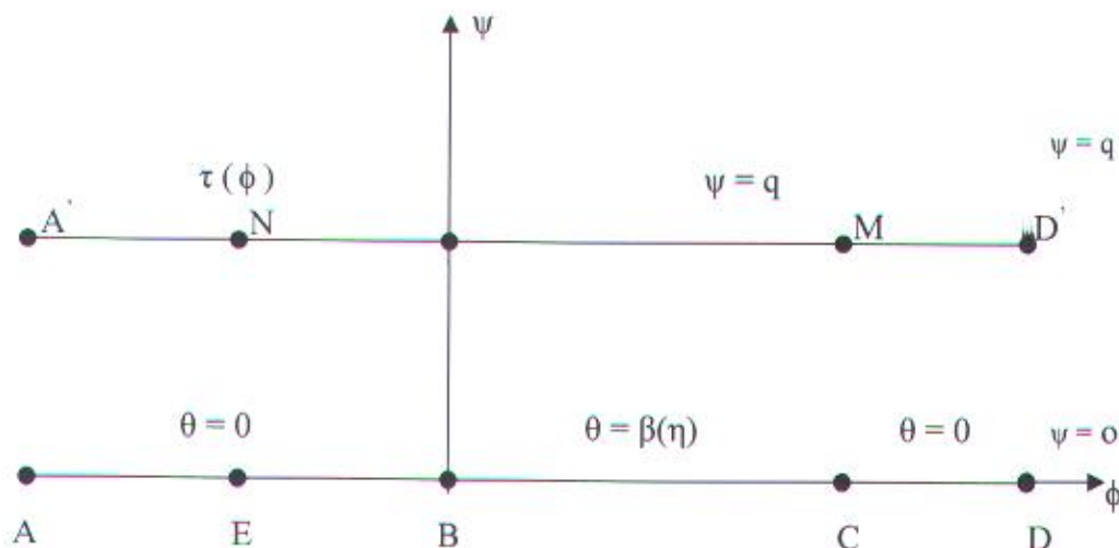
Gambar 3.2. Pemetaan bidang-Z ke bidang- \omega
