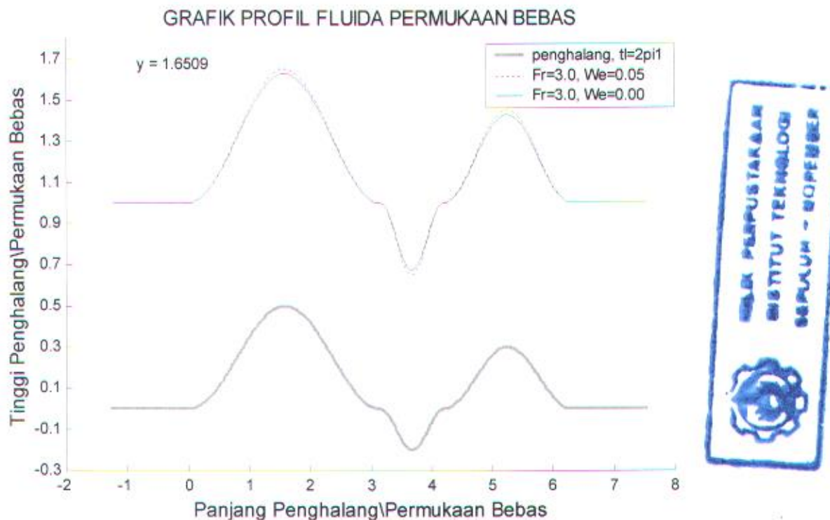
Gambar 4.3. Profil permukaan bebas dengan bilangan Fr=3.0 , dengan variasi bilangan We=0.05 , We=0.00 .
