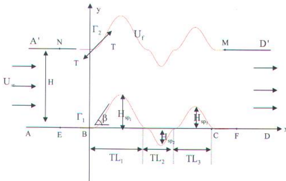
Gambar 3.1. : Bidang fisis untuk aliran di permukaan bebas di atas penghalang dipengaruhi pengaruh gravitasi dan tegangan permukaan.
