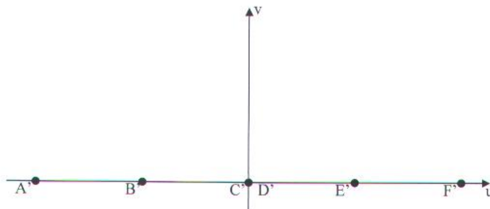
Gambar 2.2. Bidang paruh-W bagian atas
