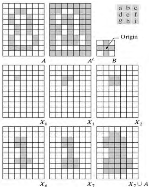
Gambar 2.19 Operasi region filling (a) Himpunan A (b) Komplement dari A (c) Structuring element B (d) Titik awal pada boundary (e)-(h) Langkah-langkah pada persamaan 2.12 (i) Hasil final yang merupakan union dari (a) dan (b)
