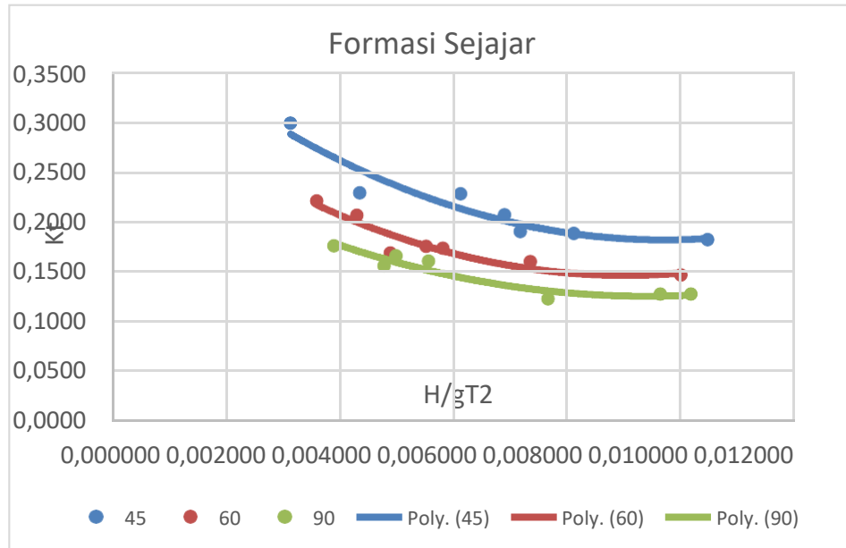
Gambar 4. 20 Grafik Pengaruh sudut terhadap Kt pada Struktur OWS yang Disusun dengan formasi sejajar
