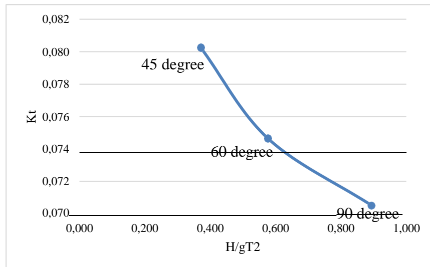
Gambar 4. 12 Koefisien transmisi formasi sejajar
