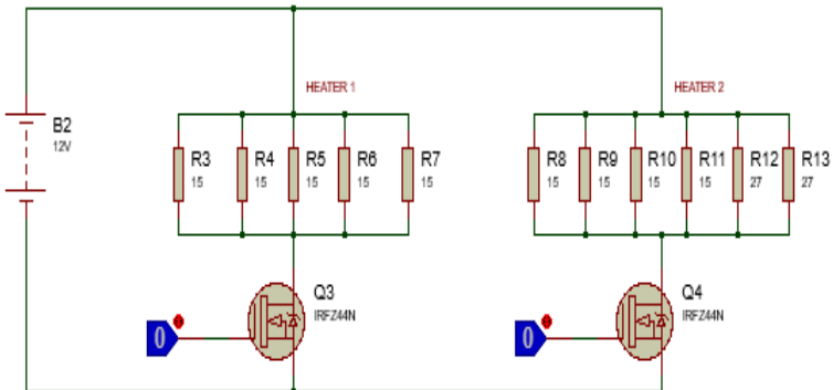
Gambar 3.3 Rangkaian Heater
