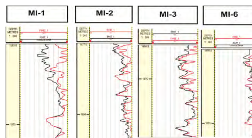
Gambar 2 Tampilan porositas keempat sumur
