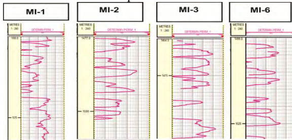
Gambar 4 Permeabilitas keempat sumur
