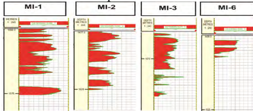
Gambar 3 Saturasi Air keempat sumur
