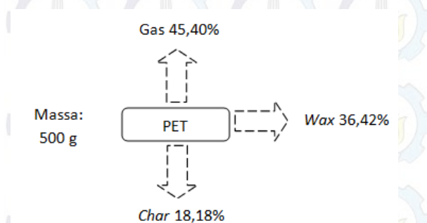
Gambar 2 Skema Pirolisis Plastik PET
