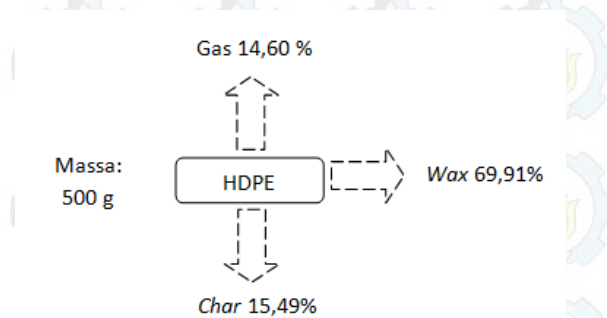
Gambar 1 Skema Pirolisis Plastik HDPE
