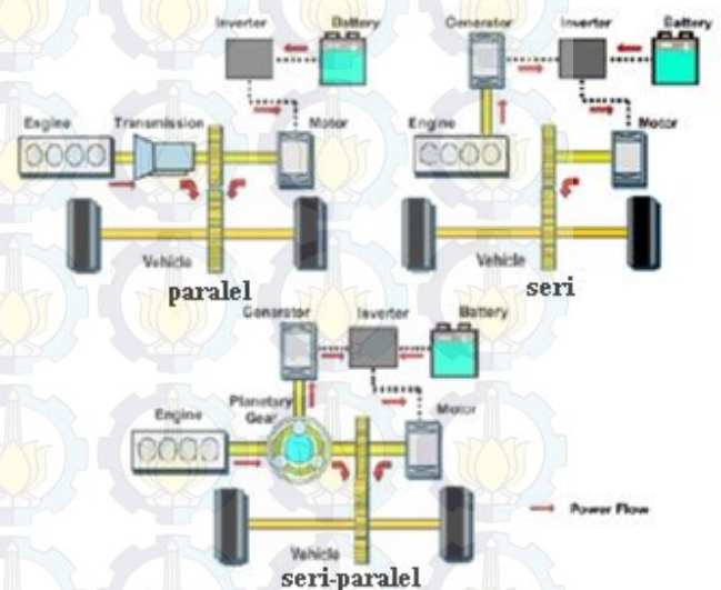
Gambar 1. Konfigurasi HEV [1]
