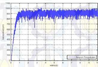
Gambar 5. Respon Kecepatan ICE dengan Beban Nominal
