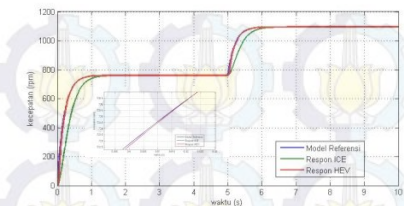
Gambar 13. Respon ICE Berbeban Dengan Bantuan Motor DC Tanpa Model Prediksi Terhadap Sinyal dengan Amplitudo Berubah
