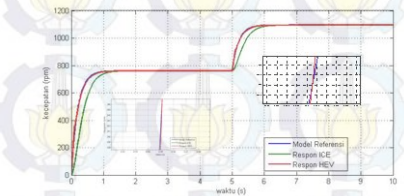
Gambar 15. Respon ICE Berbeban Dengan Bantuan Motor DC Menggunakan Model Prediksi Terhadap Sinyal dengan Amplitudo Berubah
