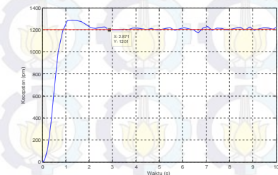
Gambar 8. Respon Kecepatan Motor DC
