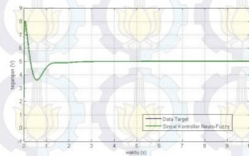
Gambar 12. Output Kontroler Neuro-Fuzzy Dengan \alpha=0,01
