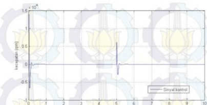
Gambar 16. Sinyal Kontrol Motor DC Menggunakan Model Prediksi Terhadap Sinyal dengan Amplitudo Berubah
