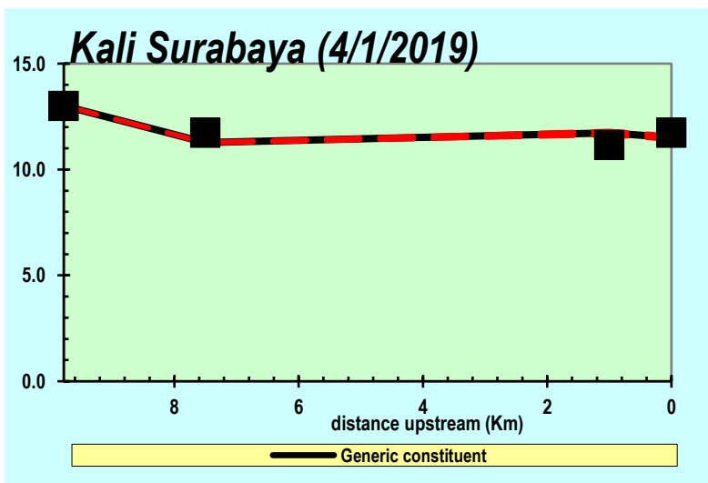
Gambar 4.7 Kalibrasi COD
