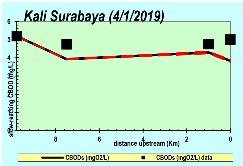
Gambar 4.6 Kalibrasi BOD
