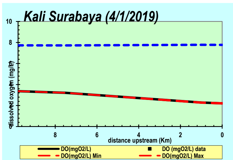
Gambar 4.13 Simulasi 2 DO
