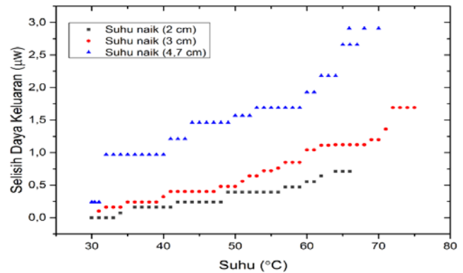
Gambar 4 Grafik Hubungan Suhu dengan Selisih Daya Keluaran pada Panjang kupasan 2 cm, 3 cm dan 4,7 cm dengan Panjang Gelombang Sumber 1310 nm untuk Suhu Naik
