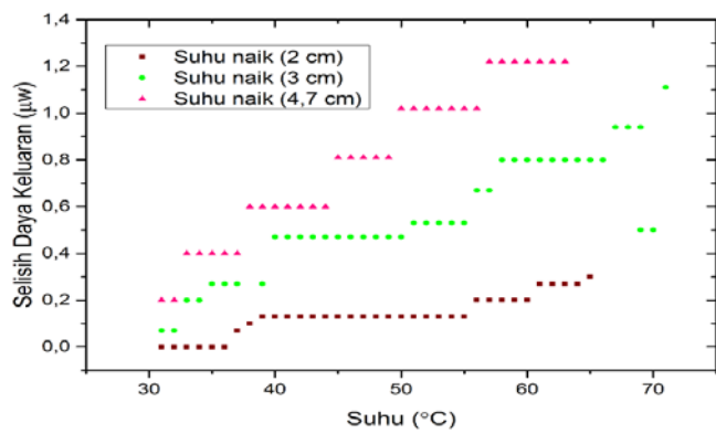
Gambar 6 Grafik Hubungan Suhu dengan Selisih Daya Keluaran pada Panjang kupasan 2 cm, 3 cm dan 4,7 cm dengan Panjang Gelombang Sumber 1550 nm untuk Suhu Naik
