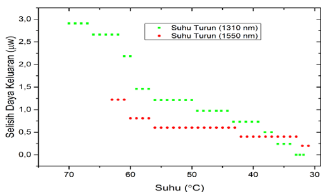
Gambar 13 Grafik Hubungan Suhu dengan Selisih Daya Keluaran pada Panjang kupasan 4,7 cm dengan panjang gelombang sumber 1310 nm dan 1550 nm untuk Suhu Turun
