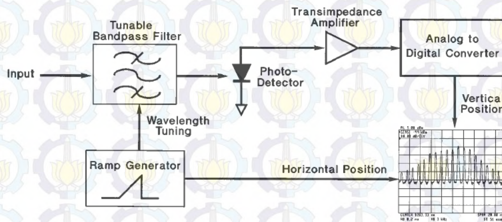
Gambar 2. 10 Diagram Blok Dasar OSA
