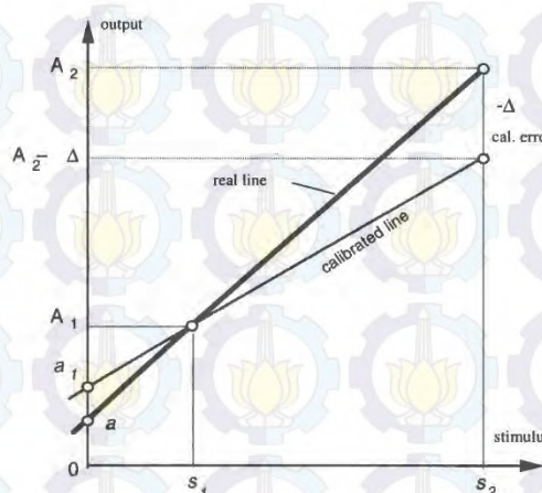
Gambar 2. 11 Penentuan Error Kalibrasi
