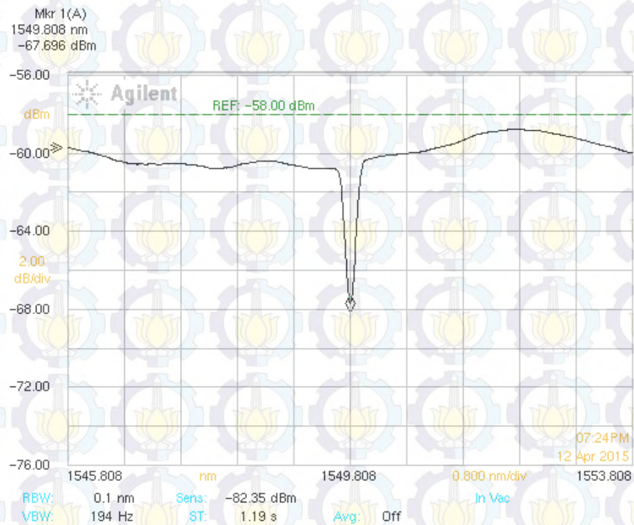
Gambar 4. 3.Spektrum Transmisi FBG C.W. 1550 \pm 0.5 nm
