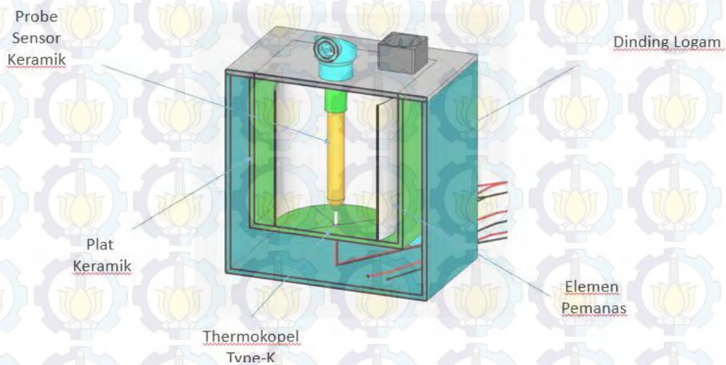
Gambar 3. 5 Desain Furnace untuk pengukuran
