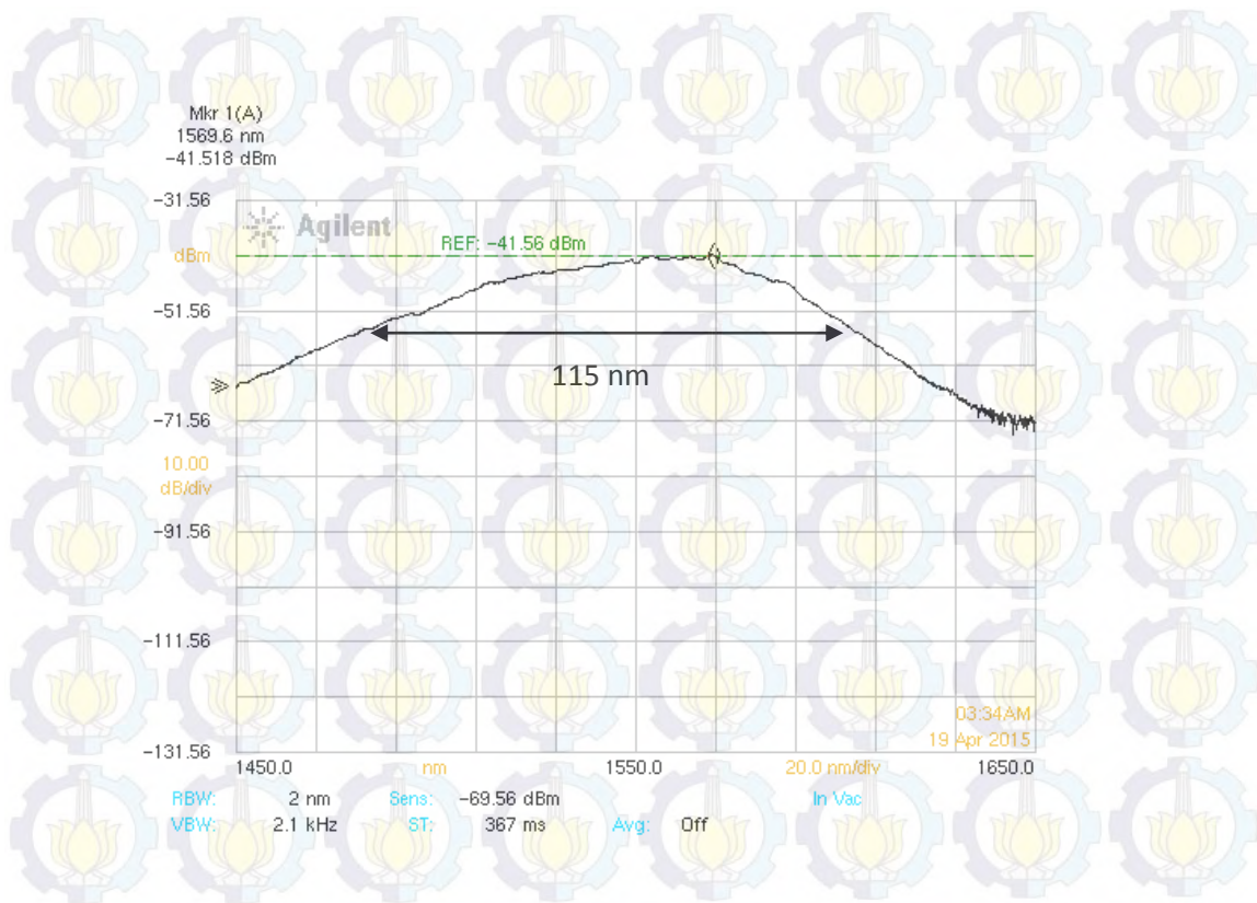
Gambar 4. 1. Interface FBG pada Optical Spectrum Analyzer (OSA agilent 86142 B)
