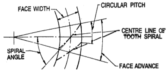
Gambar 2 Sudut spiral [1]
