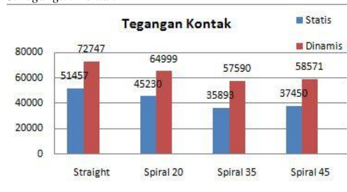
Gambar 10. Nilai Tegangan Kontak
