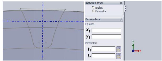
Gambar 5 sket profil gigi
