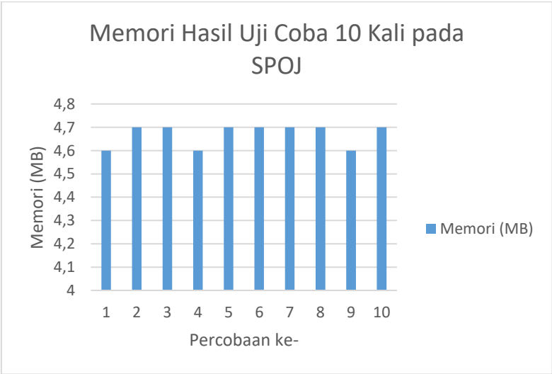
Gambar 5.4: Grafik memori hasil uji kebenaran sebanyak 10 kali pada SPOJ
