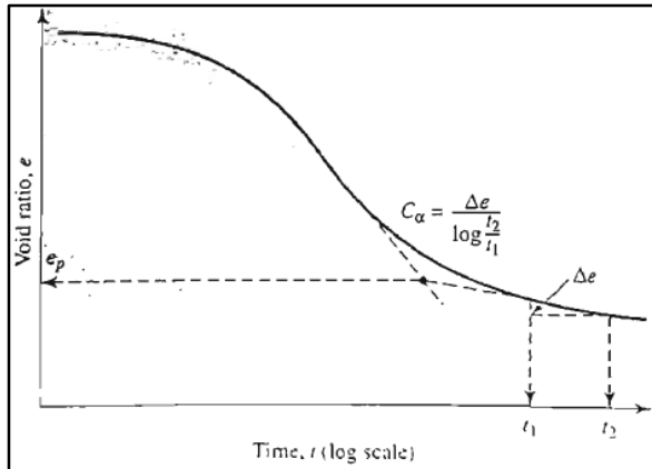
Gambar 2.4 Kurva Waktu Terjadinya Konsolidasi Sekunder
