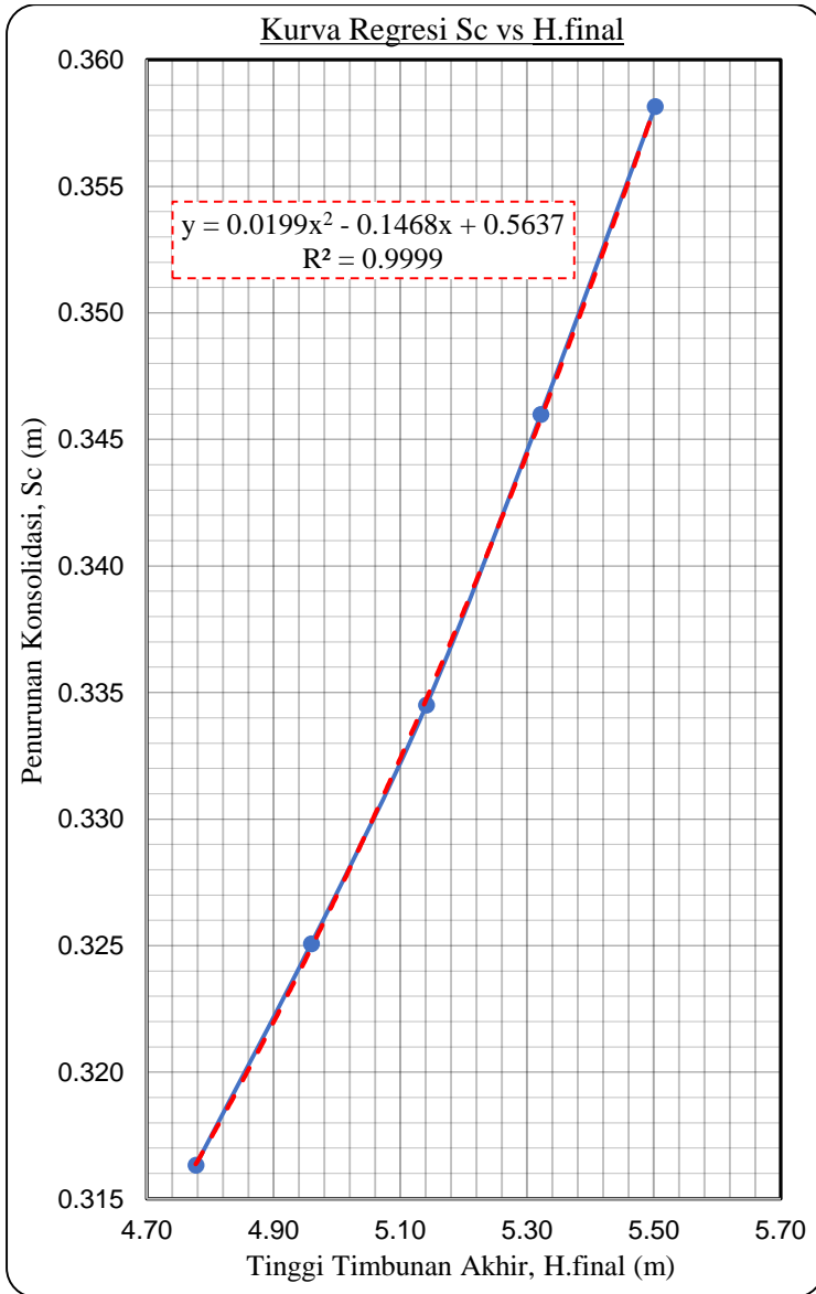
Gambar 4.7 Kurva Regresi Sc vs H.final Zona 3
