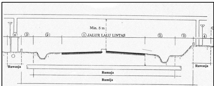
Gambar 5.1 Standar Penetapan Ruang Jalan
