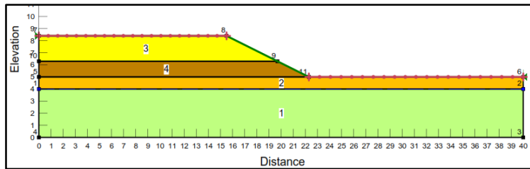
Gambar 4.18 Permodelan Awal Zona 4 Sebelum Running
