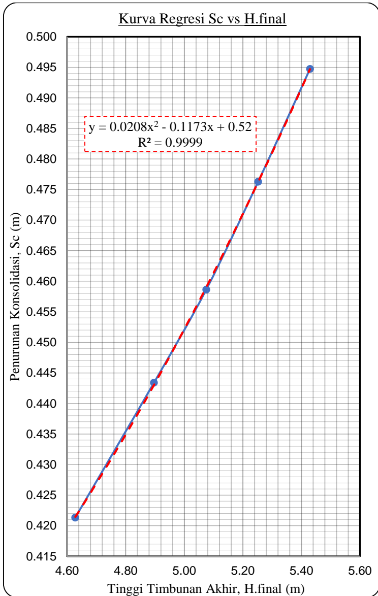
Gambar 4.5 Kurva Regresi Sc vs H.final Zona 2
