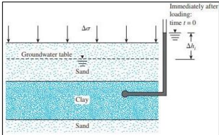
Gambar 2.1 Prinsip Konsolidasi
