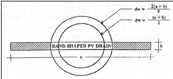
Gambar 2.6 Diameter Ekuivalen untuk PVD
