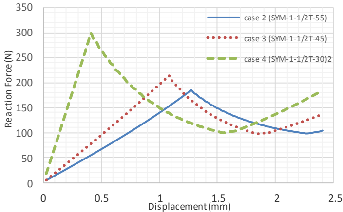
Gambar 4 Pengaruh Panjang Initial Crack
