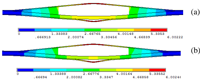
Gambar 11 penampang displacement saat distribusi tegangan 2 buah (a) symmetric , dan; (b) unsymmetric .
