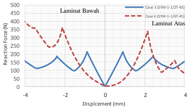
Gambar 6 Lokasi Initial Crack panjang a = 45 mm saat 1/2 t dan 1/6 t.
