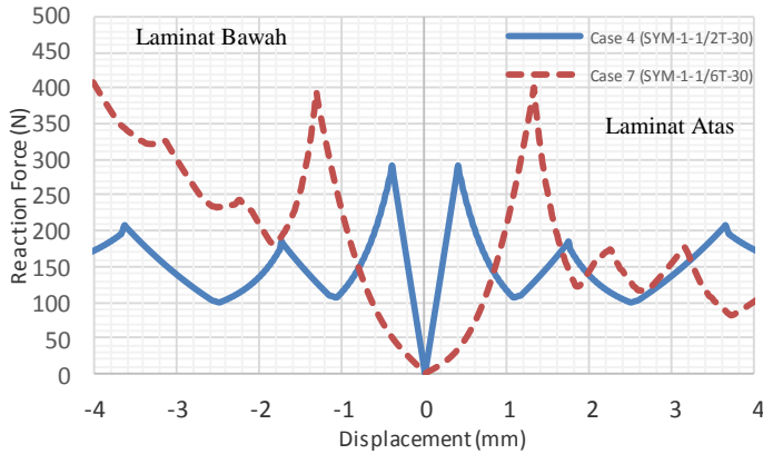
Gambar 7 Lokasi Initial Crack panjang a = 30 mm saat 1/2 t dan 1/6 t
