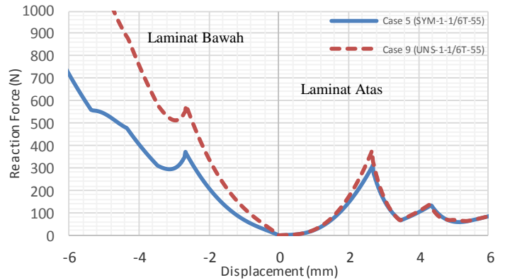
Gambar 9 Konfigurasi Lay-up saat 1/6 t
