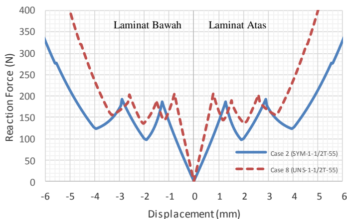
Gambar 8 Konfigurasi Lay-up saat 1/2 t
