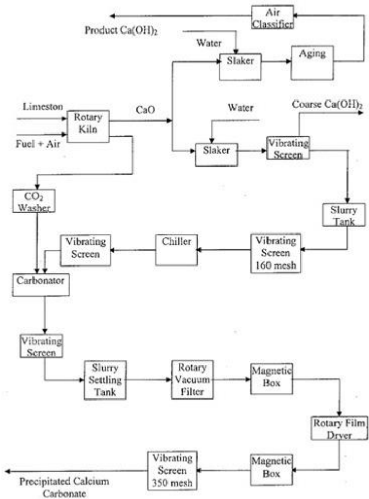
Gambar III.4 Pembuatan PCC pada Plant Dhaka (Shahinoor, 2007)
