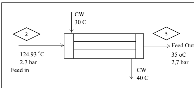
IV.18 Neraca Energi Cooler (E-113)
