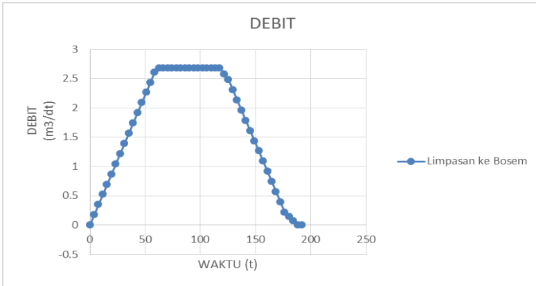
Gambar 4.19. Grafik debit limpasan dari saluran Baru dan Sambikerep ke bosem ( t_c < t_d ).
