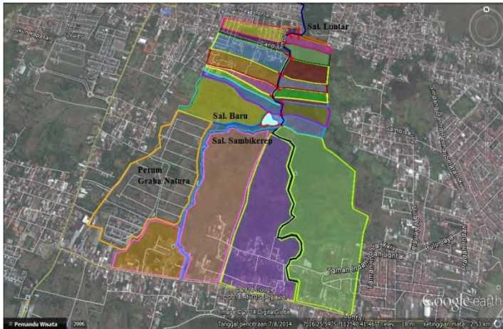
Gambar 4.25. Das saluran Lontar.
