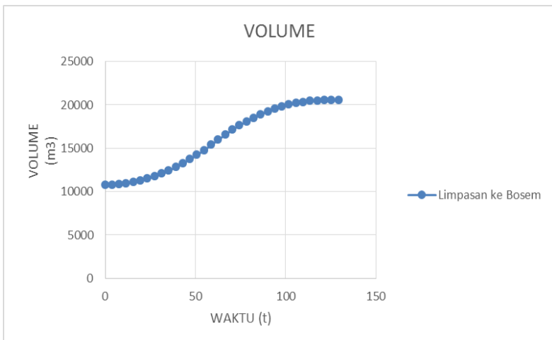
Gambar 4.18. Grafik volume limpasan dari saluran Baru dan Sambikerep ke bosem ( t_c = t_d ).
