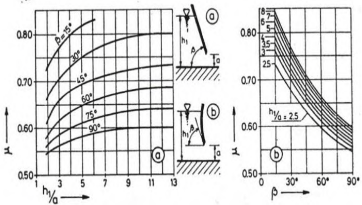
Gambar 2.10 Koefisien debit K_d masuk permukaan pintu datar atau lengkung
