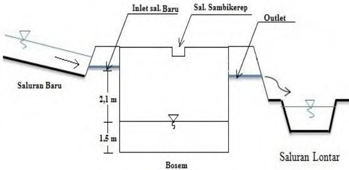
Gambar 4.16. Gambar kondisi penampang bosem pada saat musim hujan.
