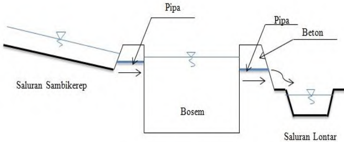
Gambar 2.3 Kondisi kolam tampungan (bosem kecil)
