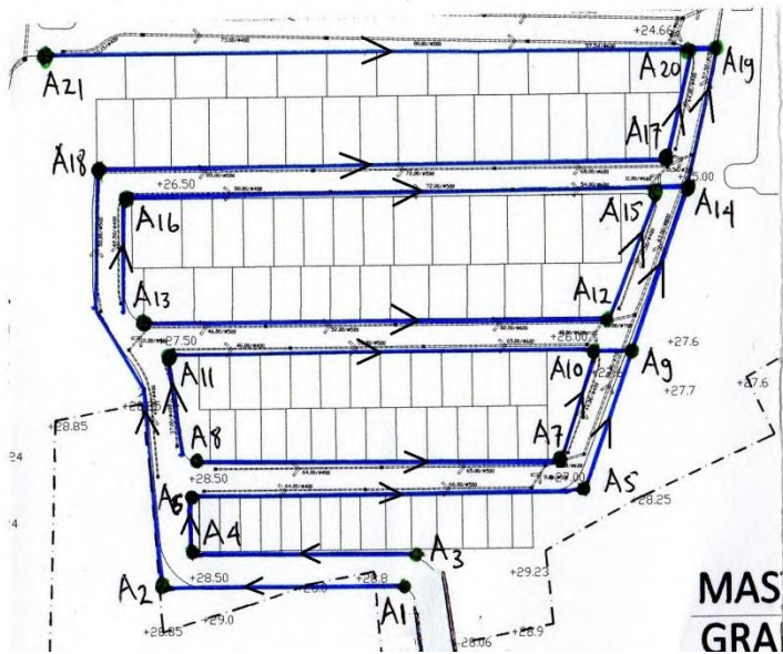
Gambar 4.12. Rencana jaringan drainase pada sebagian Site Plan.
