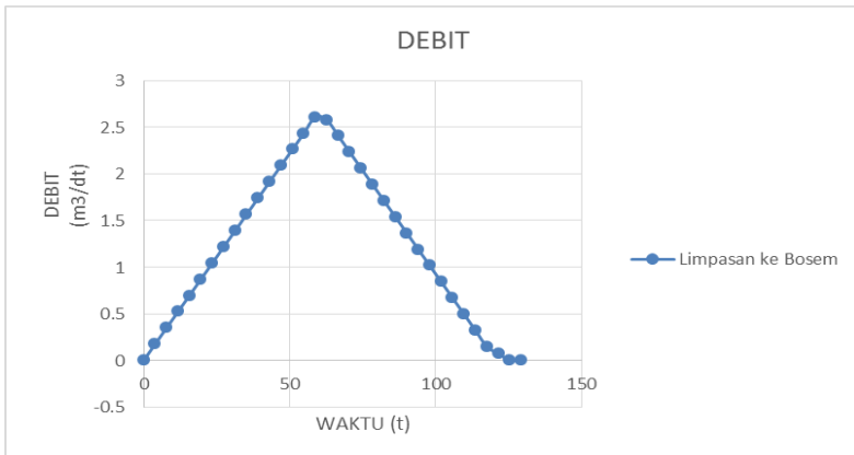
Gambar 4.17. Grafik debit limpasan dari saluran Baru dan Sambikerep ke bosem ( t_c = t_d ).
