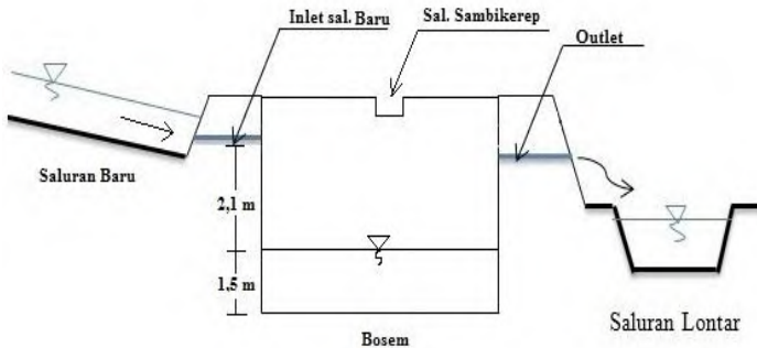
Gambar 4.10. Gambar kondisi penampang bosem pada saat musim hujan
