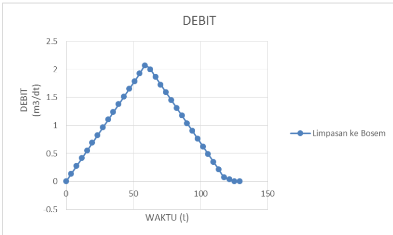
Gambar 4.21. Grafik debit limpasan dari saluran Baru dan Sambikerep ke Bosem ( t_c = t_d ).
