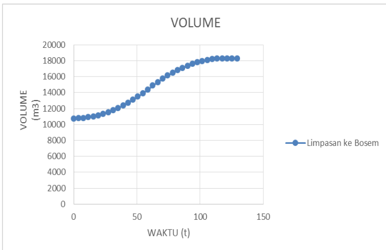
Gambar 4.22. Grafik volume limpasan dari saluran Baru dan Sambikerep ke Bosem ( t_c = t_d ).
