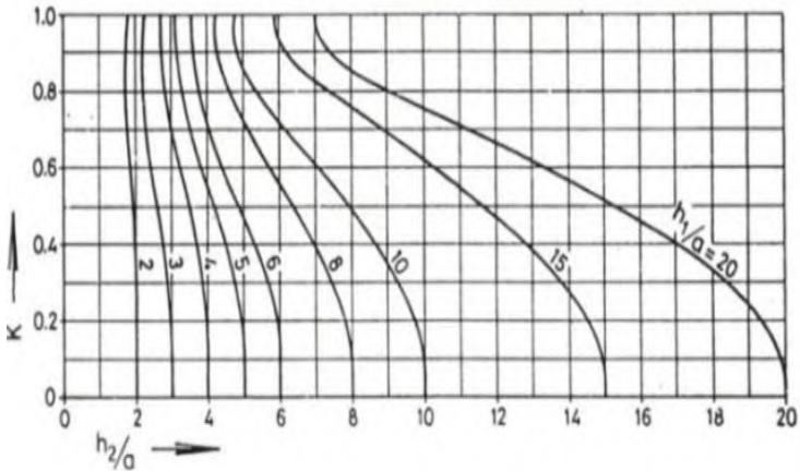
Gambar 2.9 Grafik Koefisien K untuk aliran tenggelam
