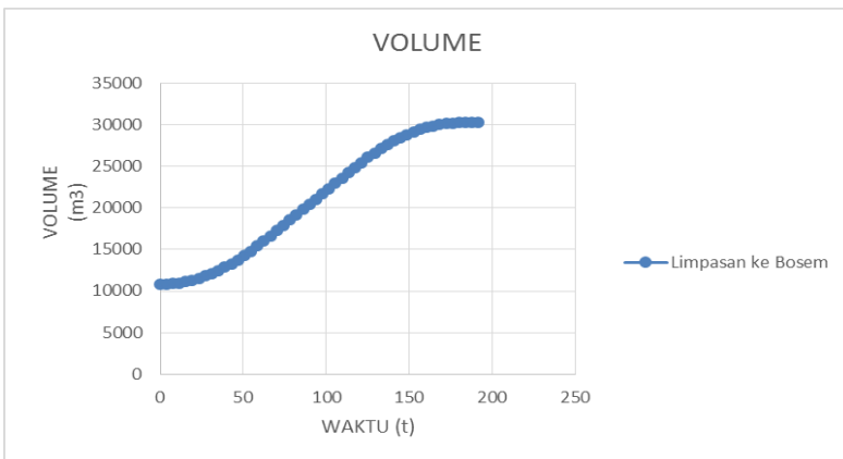
Gambar 4.20. Grafik volume limpasan dari saluran Baru dan Sambikerep ke bosem ( t_c < t_d ).
