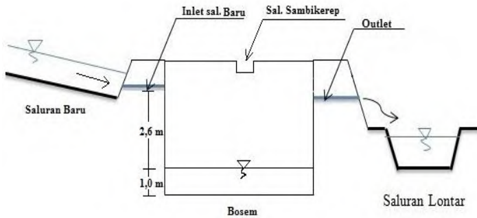
Gambar 4.9. Gambar kondisi penampang bosem pada saat musim kemarau
