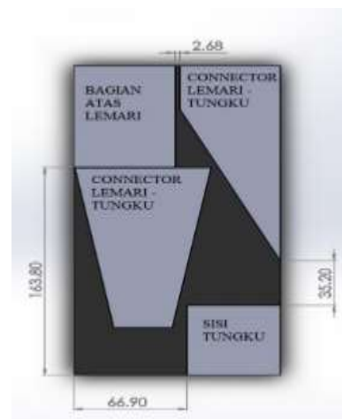
Gambar 5.0 Plat 3
