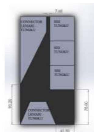
Gambar 5.1 Plat 4
