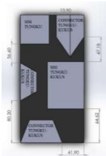
Gambar 5.2 Plat 5
