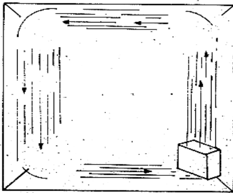
Gambar 3.4. Perpindahan panas secara konveksi
