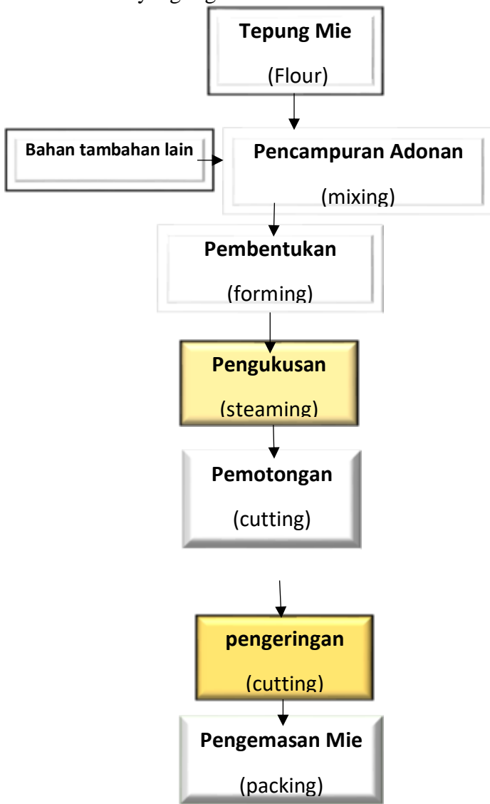
Gambar 2.1. Diagram alir proses produksi
