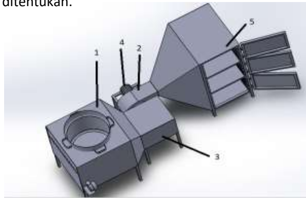
Gambar 4.2 Bagian Pengeringan Mie
