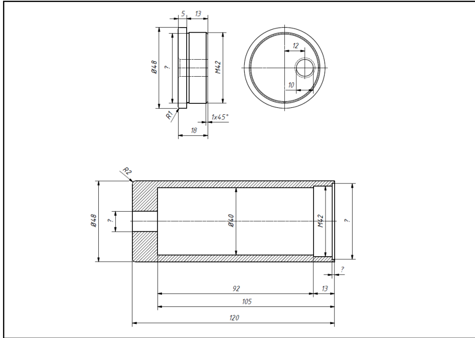
Gambar Teknik Alat Jet Clean 100 ml
