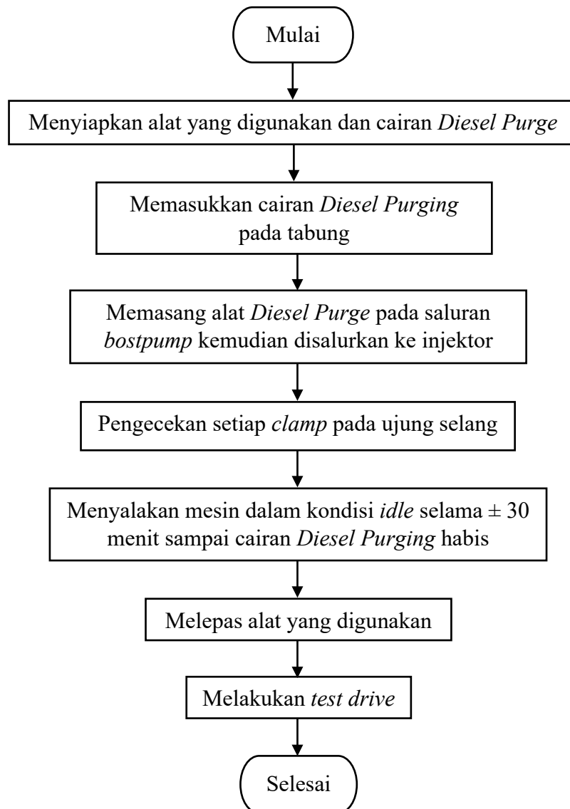
Gambar 5. 10 Diagram Alir Proses Diesel Purging pada Mobil
