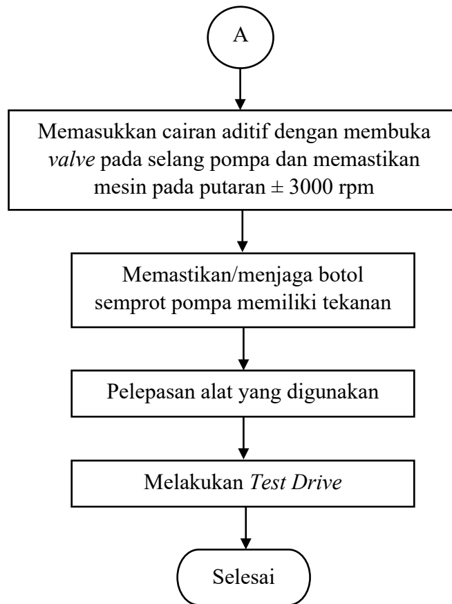
Gambar 5. 7 Diagram Alir Proses Catalytic System Cleaner pada Mobil
