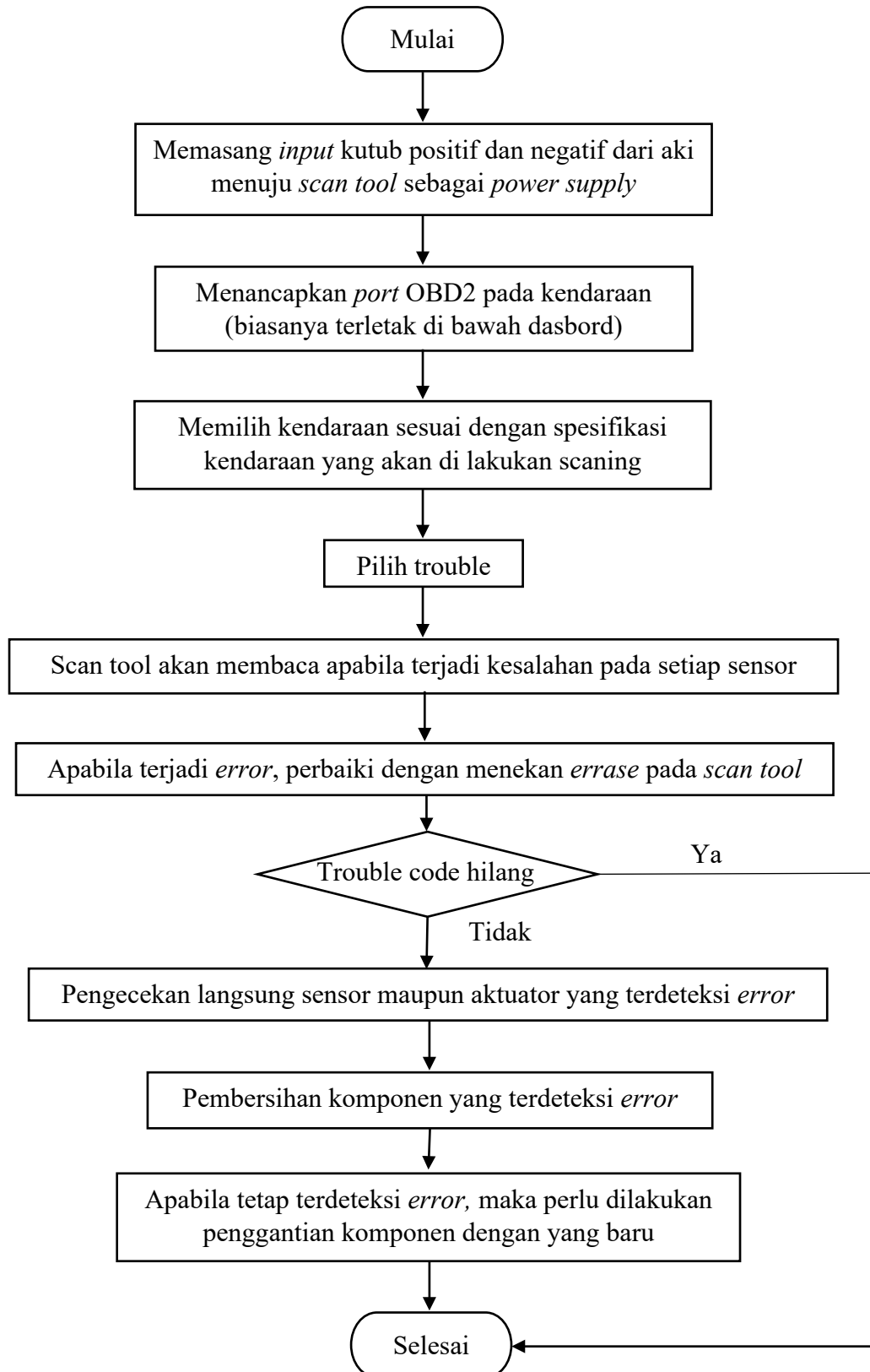
Gambar 5. 8 Diagram Alir Proses Scan pada Mobil
