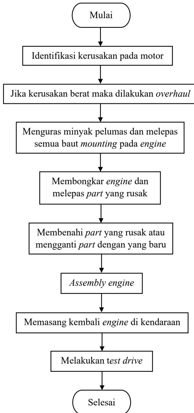
Gambar 5. 15 Diagram Alir Overhaul pada Motor
