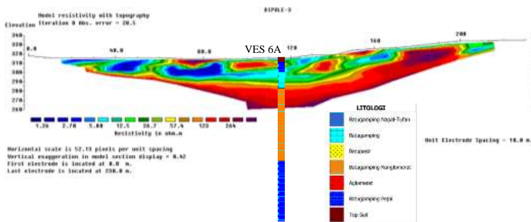
Gambar 4. 27 Validasi data VES 6A menggunakan data geolistrik 2D lintasan Dipole-3 berdasarkan perbedaan litologi.
