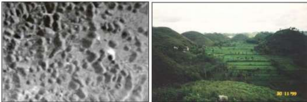
Gambar 2.4 Kenampakan Kegelkarst Gunungsewu dari foto udara dan lapangan (Sumber : Haryono & Adji, 2004).
