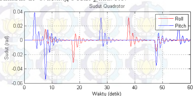
Gambar 3. Sudut Roll dan Pitch untuk Gerak Quadrotor
