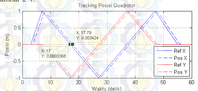
Gambar 2. Tracking Posisi Quadrotor
