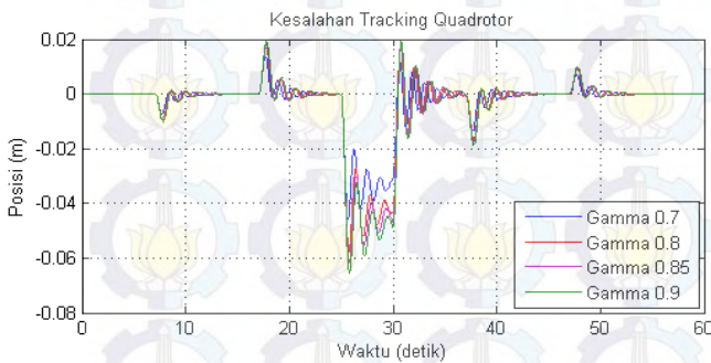
Gambar 9. Kesalahan Posisi Y
