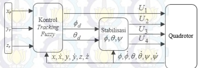
Gambar 1. Arsitektur Sistem Kontrol untuk Quadrotor
