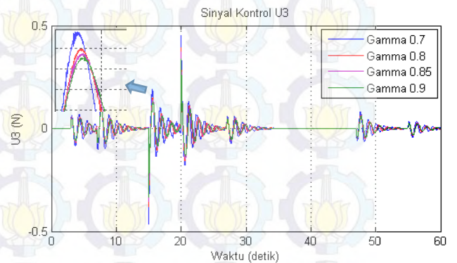
Gambar 7. Sinyal Kontrol U3 untuk Gerak Sumbu X
