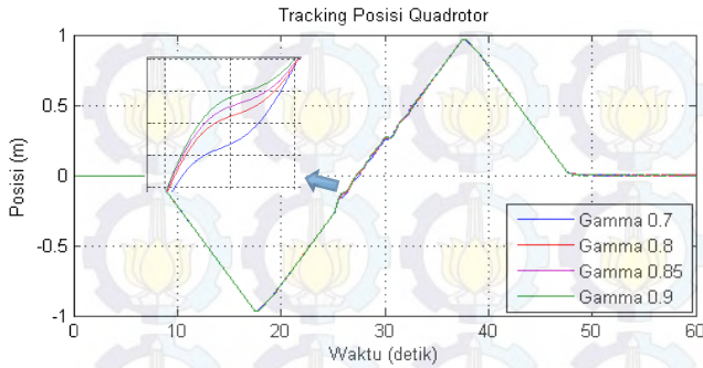
Gambar 8. Perbandingan Posisi Quadrotor dengan Variasi \gamma
